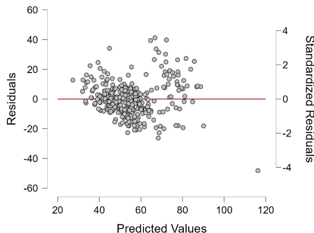
Gambar 2. Uji Heteroskesdaktisitas
