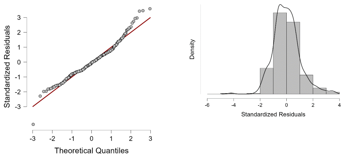
Gambar 1. Uji Normalitas
