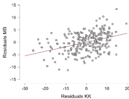
Gambar 2. Uji Linieritas
