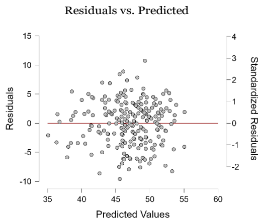
Gambar 4. Uji Homoskedastisitas
