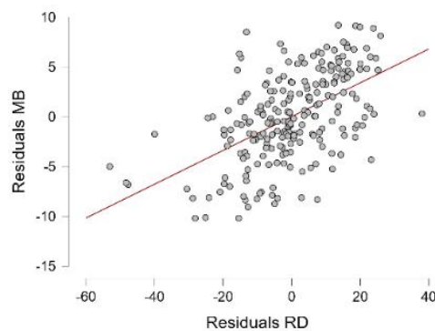
Gambar 3. Uji Linieritas
