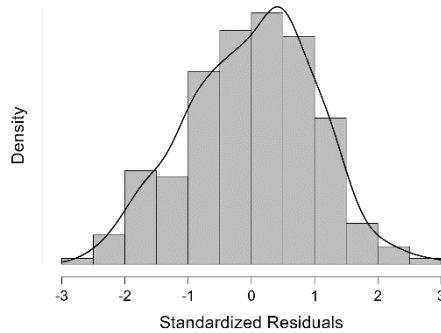
Gambar 1. Uji Normalitas
