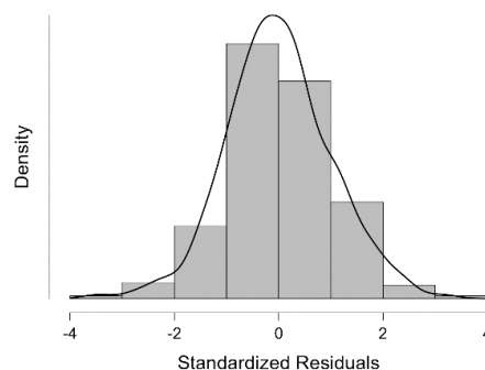
Gambar 1. Uji Normalitas
