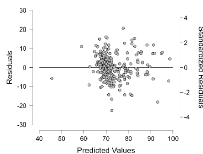
Gambar 4. Uji Homoskedastisitas
