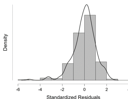
Gambar 1. Uji Normalitas
