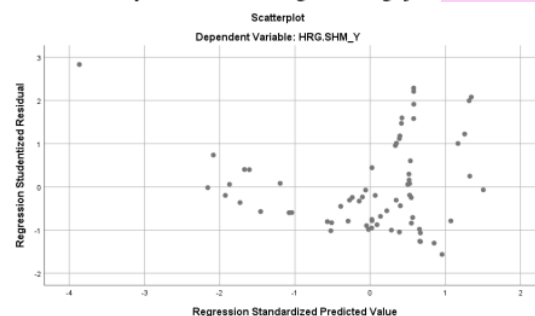
Gambar 1 Uji Heterokedastisitas
