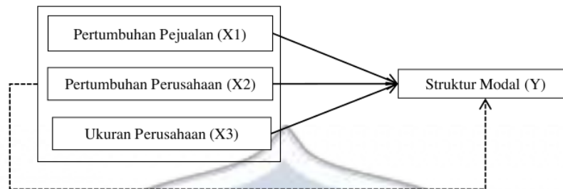
Gambar 1. Kerangka Konseptual
