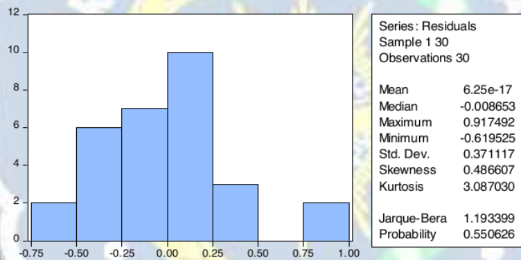
Gambar 2. Uji Normalitas
