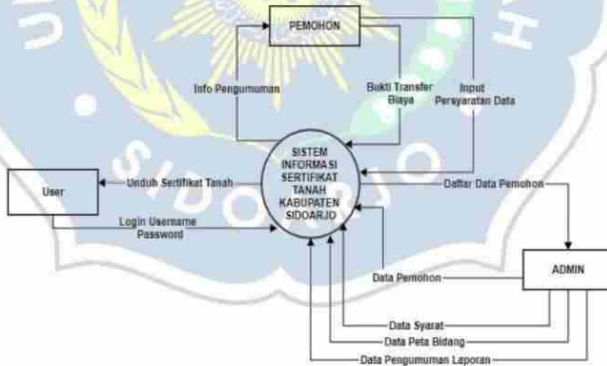
Gambar.3 Data Flow Diagram Sistem Dapat dilihat dari Data Flow Diagram Diatas Bahwa Sistem Informasi Pembuatan Tanah pada Kantor Pertanahan Kabupaten Sidoarjo
